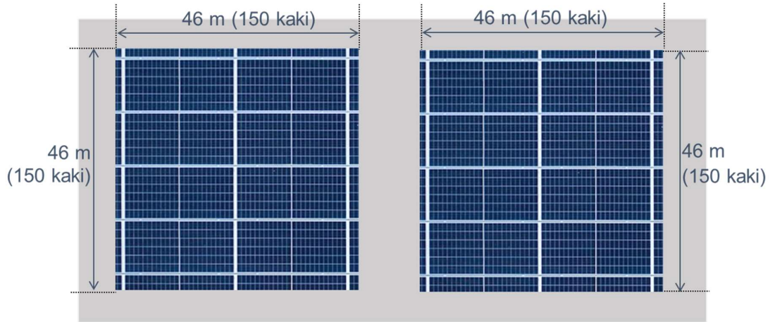
Rajah 15 : Ilustrasi tatasusunan modul fotovoltaik hendaklah tidak melebihi 46m x 46m
